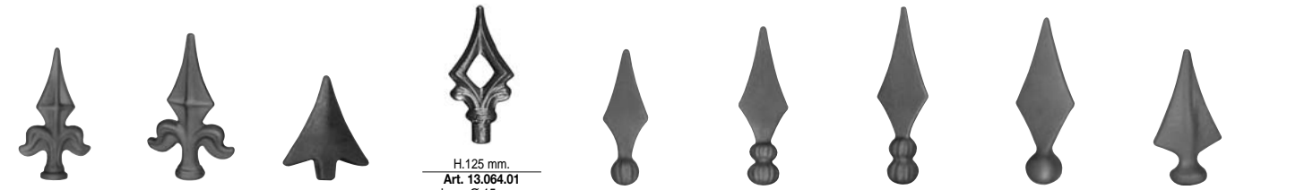
H.115 X L. 58 mm. Art. 13.060 Ø 20 H.140 X L. 70 mm. Art. 13.061 Ø 26 H.70 X L. 60 mm. Art. 13.063 12 H.125 mm. Art. 13.064.01 base Ø 15 mm. H.100 mm. Art. 13.064.02 base Ø 12 mm. H.125 X L. 40 mm. Art. 13.071 Ø 25 H.160 X L. 50 mm. Art. 13.073 Ø 30 H.190 X L. 55 mm. Art. 13.074 Ø 32 H.175 X L. 60 mm. Art. 13.075 Ø 35 H.125 X L. 60 mm. Art. 13.077 Ø 32
