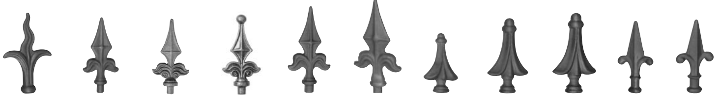
H.140 X L. 90 mm. Art. 13.051 Ø 30 H.130 X L. 60 mm. Art. 13.052 Ø 12 H.130 X L. 60 mm. Art. 13.052.1 Ø 12 H.135 X L. 60 mm. Art. 13.052.3 Ø 12 H.155 X L. 70 mm. Art. 13.053 Ø 17 H.190 X L. 95 mm. Art. 13.054 Ø 20 H.80 X L. 45 mm. Art. 13.055 Ø 20 H.125 X L. 65 mm. Art. 13.056 Ø 25 H.140 X L. 80 mm. Art. 13.057 Ø 38 H.120 X L. 55 mm. Art. 13.058 Ø 20 H.135 X L. 65 mm. Art. 13.059 Ø 25
