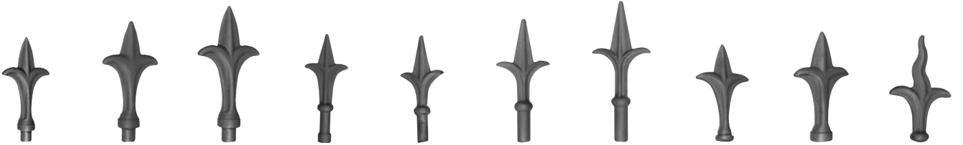
H.125 X L. 60 mm. Art. 13.041 Ø 13 H.155 X L. 70 mm. Art. 13.042 Ø 17 H.190 X L. 90 mm. Art. 13.043 Ø 20 H.130 X L. 50 mm. Art. 13.044 Ø 15 H.130 X L. 53 mm. Art. 13.045 Ø 13 H.160 X L. 65 mm. Art. 13.046 Ø 17 H.200 X L. 85 mm. Art. 13.047 Ø 20 H.110 X L. 60 mm. Art. 13.048 Ø 20 H.135 X L. 70 mm. Art. 13.049 Ø 26 H.130 X L. 70 mm. Art. 13.050 Ø 20
